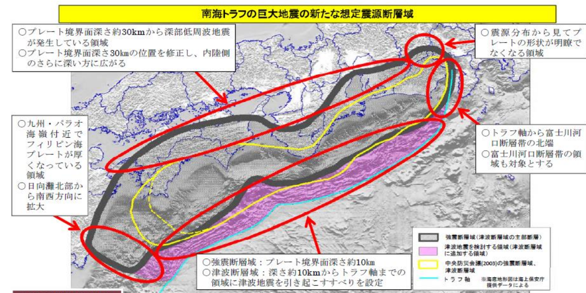
南海トラフ巨大地震の想定震源断層域
